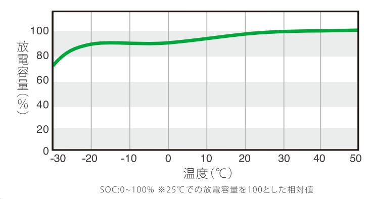
■ 放電容量温度特性
