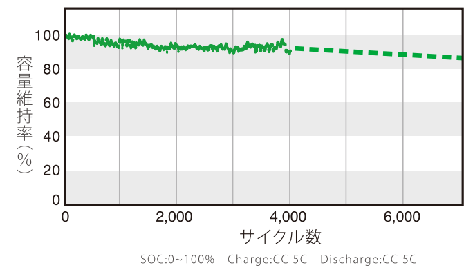
■ サイクル寿命特性(充電5C/放電5C:25℃)
