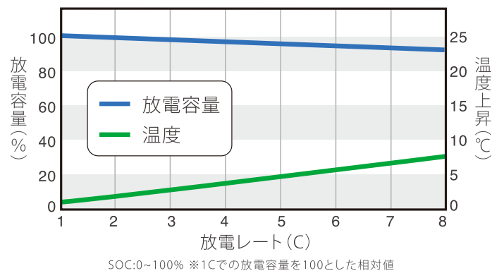
■ 放電レート特性
