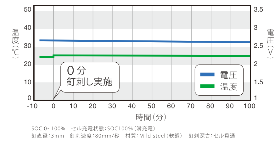
■ 釘刺試験(SAE J2464)
