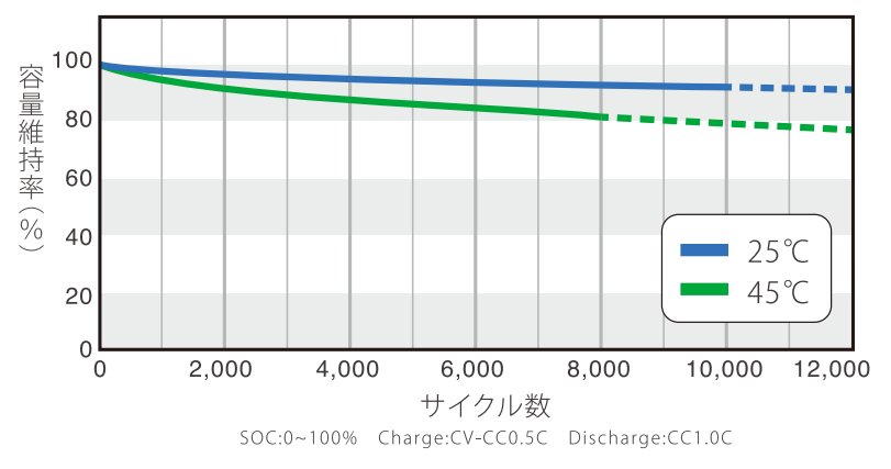
■ サイクル寿命特性(充電0.5C/放電1C)
