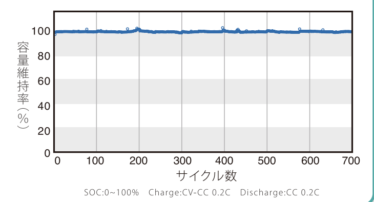
■ サイクル寿命特性(充電0.2C/放電0.2C:-20℃)
